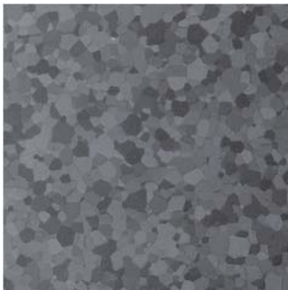
Y 2 O 3 セラミックスの微細組織 Microstructure of Y 2 O 3 ceramics
